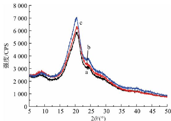
图 3 样品的 X 射线粉末衍射图 a 为纯丝绸; b 为 P50 水溶性聚合物 A 处理丝绸; c 为 P80 水溶性聚合物 A 处理丝绸
