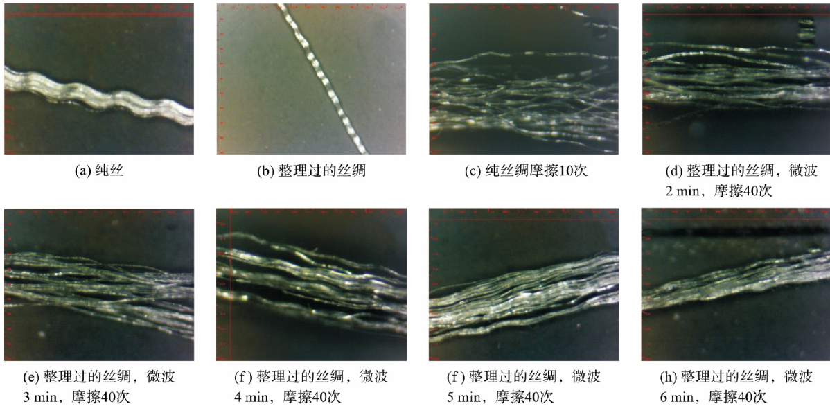
图 4 摩擦后单丝束形貌变化
