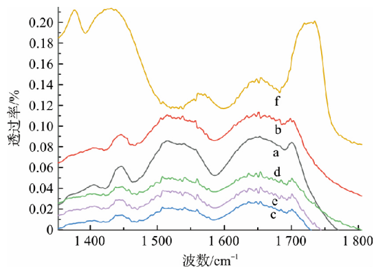
图 2 样品的红外吸收光谱图 a 为纯丝绸; b 为纯丝绸, 微波(P50) 4 min; c 为水溶性聚合物 A 整理丝绸, 微波(P50) 4 min; d 为水溶性聚合物 A 整理丝绸, 微波(P50) 5 min; e 为水溶性聚合物 A 整理丝绸, 微波(P50) 6 min; f 为水溶性聚合物 A 薄膜
